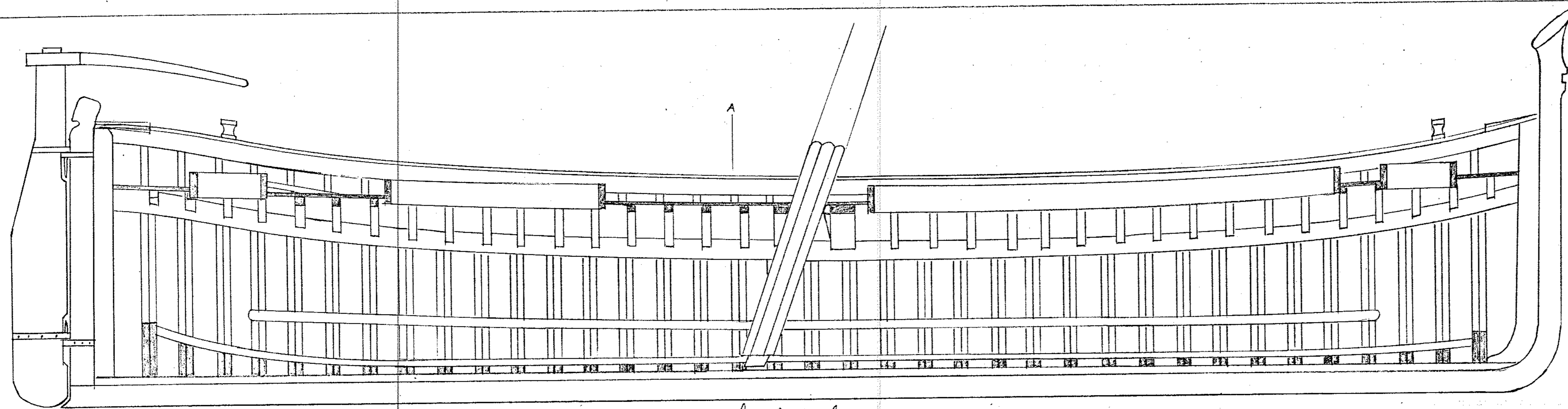
secció longitudinal
