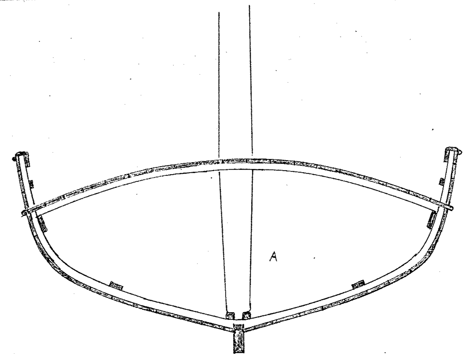
secció A
